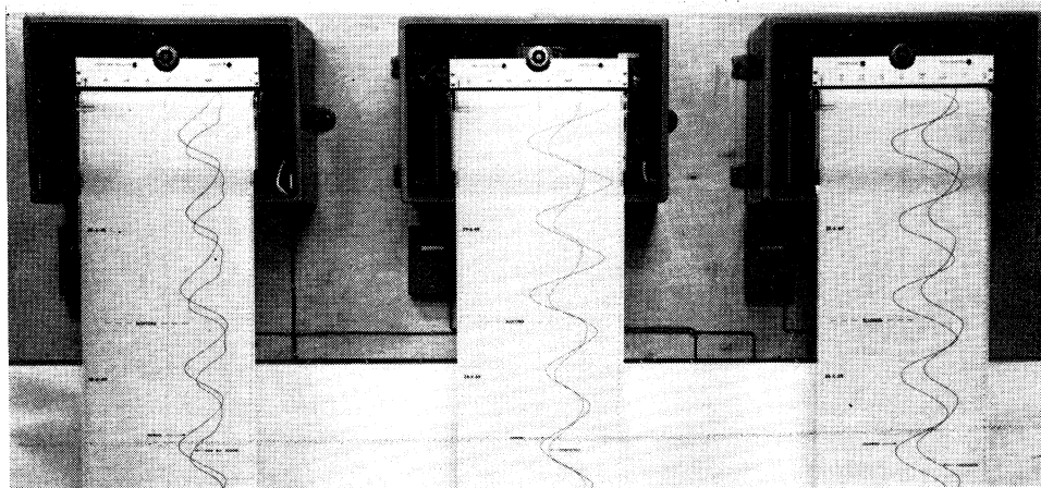
Registratie in de Deltar-zaal van het verticaal getij in verschillende peilschaalstations
