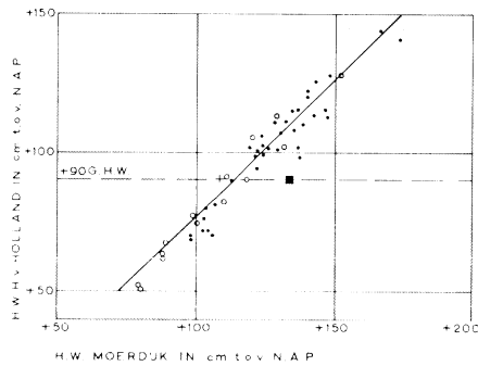
7-8. Correlatie tussen de registraties van de H.W.- en L.W.-standen in de stations Tiengemeten en Moerdijk enerzijds en het station Hoek van Holland anderzijds
