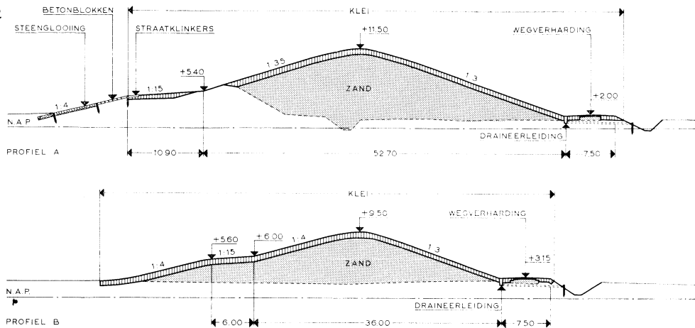
Dwarsprofielen A en B
