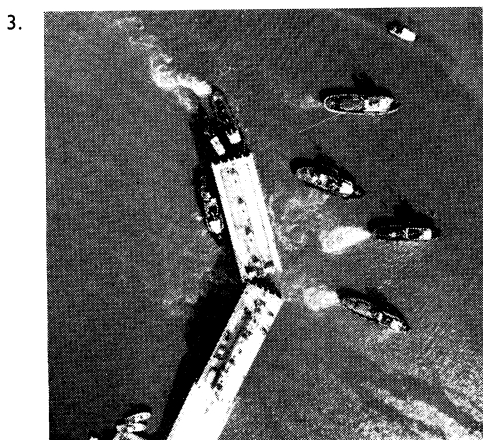
Sleepbootmanoeuvres bij het plaatsen van een doorlaatcaisson
