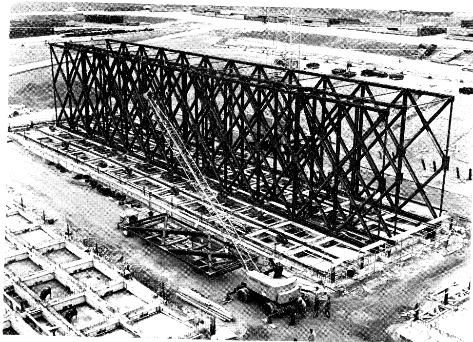
Opbouw van een caisson in het bouwdoek te Nieuw-Bommenede
