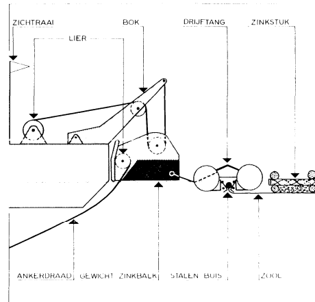
Schematische voorstelling van de werking van de drijftang
