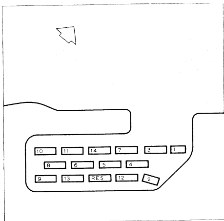
Plattegrond van het bouwdok met de caissons. De caissons zijn genummerd naar de volgorde van uitvaren
