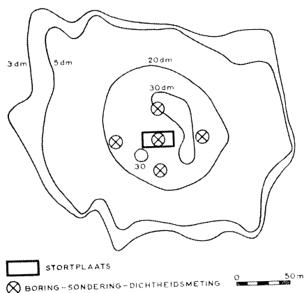
Overzicht van de stortplaats met de dikte van de laag geklapt zand
