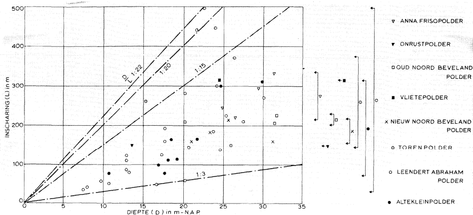
Waargenomen gemiddelde taludhellingen na een oeverval ter plaatse van enkele polders op Noord-Beveland
