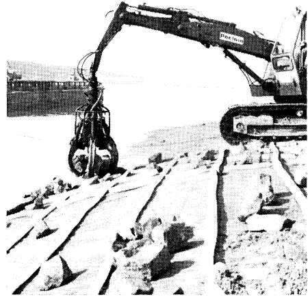
Aanbrengen van de bestorting op een kraagstuk van samengesteld kunststofweefsel
