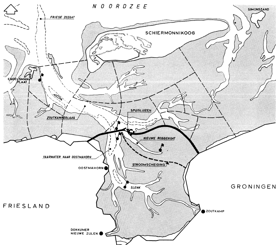
Fig. 1. De stroomgeulen in het Lauwerszeegebied. Voor de berekeningen werd het gebied schematisch ingedeeld in vakken
