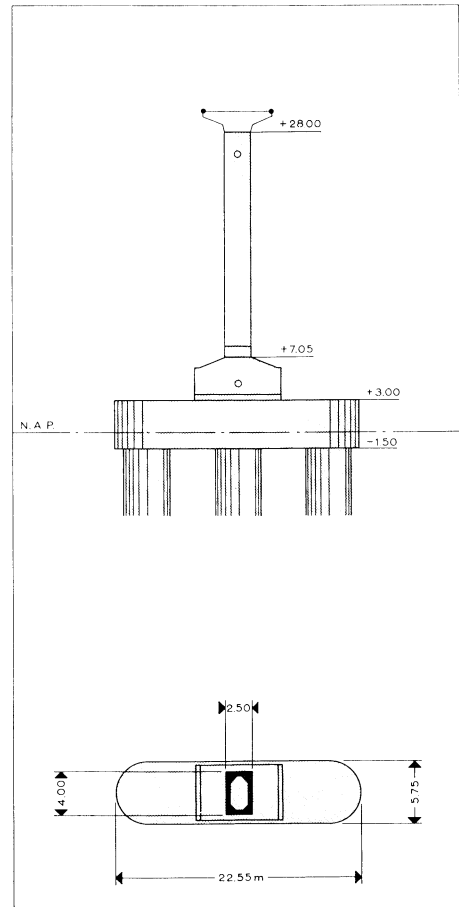
Voor- en bovenaanzicht van een rivierpyloon
