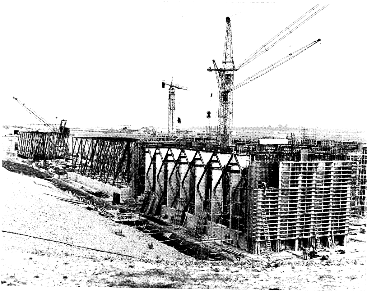
De bouw van de doorlaatcaissons bij het Volkerak; foto van september 1967
