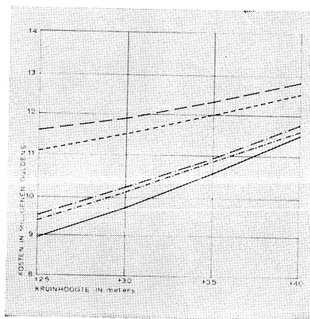
Fig. 7. Kosten van de opbouw en van herstel van schade aan de dam. De lijnen beduiden, van boven naar beneden:
