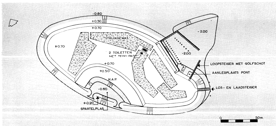
Plattegrond van de Arneplaat
