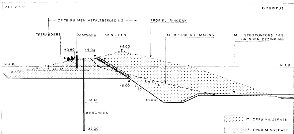
Doorsnede van de ringdijk aan de zeezijde van de bouwput met de fasen van de opruiming en de toegepaste werkwijze
