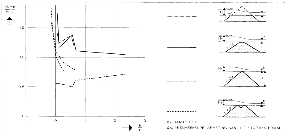
Fig. 1. Invloed van het damprofiel op de stabiliteit van het stortmateriaal
