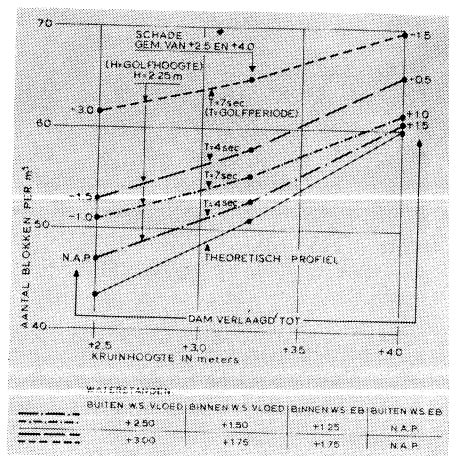
Fig. 6. Benodigd aantal betonblokken voor het opbouwen van de dam en voor herstel van schade bij stormen met een overschrijdingsfrequentie van 0,01 (bovenste twee lijnen) en 0,1 (de twee lijnen daaronder) per zomerhalfjaar
