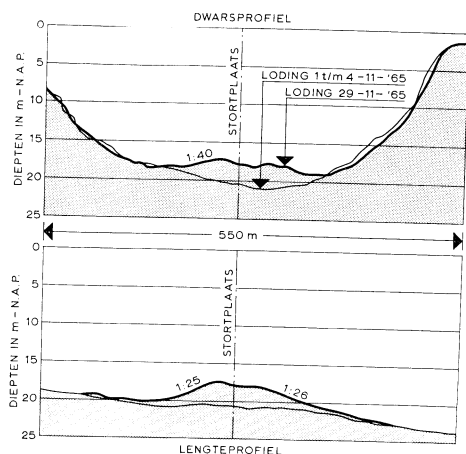
Profielen van het geklapte zand
