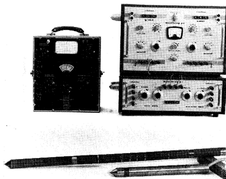
Apparatuur voor sondering en dichtheidsmeting in het terrein
