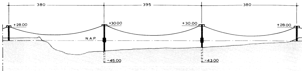
Schema van de kabeloverspanning van Schouwen (links) naar de Middelplaat
