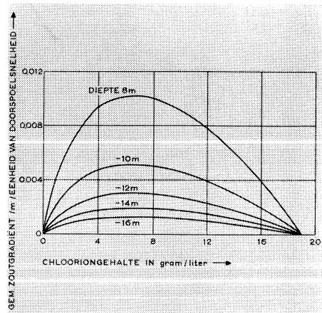
Fig. 13. De zoutgraad in gram chloorion per liter per meter lengte en per eenheid van gemiddelde ebsnelheid als functie van de diepte en het lokale gemiddelde van het chlooriongehalte tijdens de laagwaterkentering
