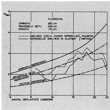
Fig. 2. Komberging van het gebied, als functie van de waterstand
