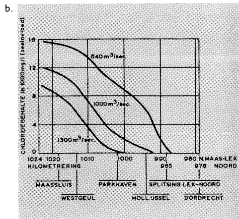
Fig. 26. a en b. Toekomstige zoutverdeling op de verondiepte Rotterdamse Waterweg bij Rijnafvoeren van 640, 1000 en 1300 m³ per seconde bij laagwaterkentering (a) en hoogwaterkentering (b)
