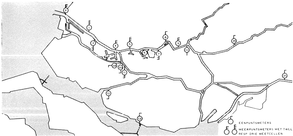
Opstelling van registerende zoutmeters langs de Nieuwe Waterweg, de Nieuwe Maas en de Oude Maas
