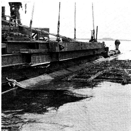
2 Verbinding van een zinkstuk met zool aan de zinkbuis; er is een overstekend zoolgedeelte voor de overlap
