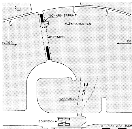
Overzicht van het sluitgat en het bouwdok in het Volkerak
