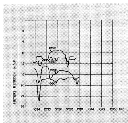
Fig. 12. Verloop van de waterdiepte in de mond van de Nieuwe Waterweg in verschillende jaren
