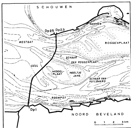
Tracé van de dam door de Oosterschelde
