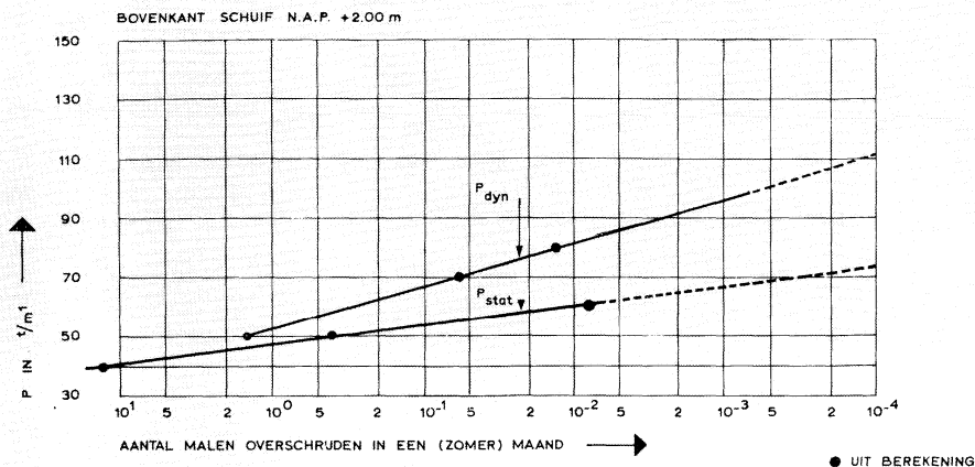
Frequentielijnen van de quasi-statische en de dynamische belastingen op de caissons
