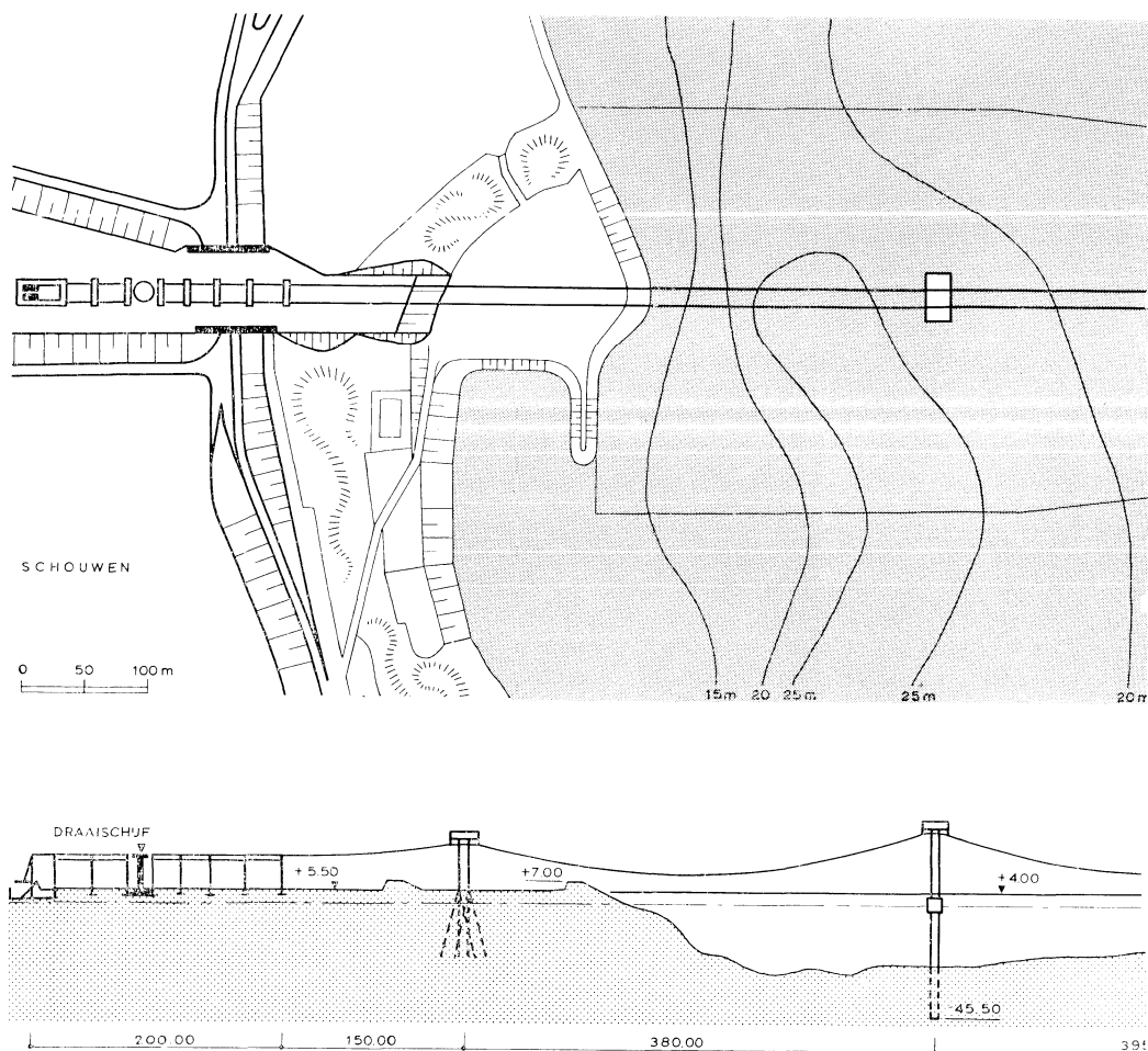
Bovenaanzicht en dwarsdoorsnede van de ontworpen kabelbaan over het Brouwershavensche Gat
