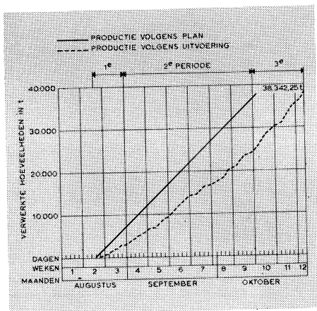
Productiegrafiek
