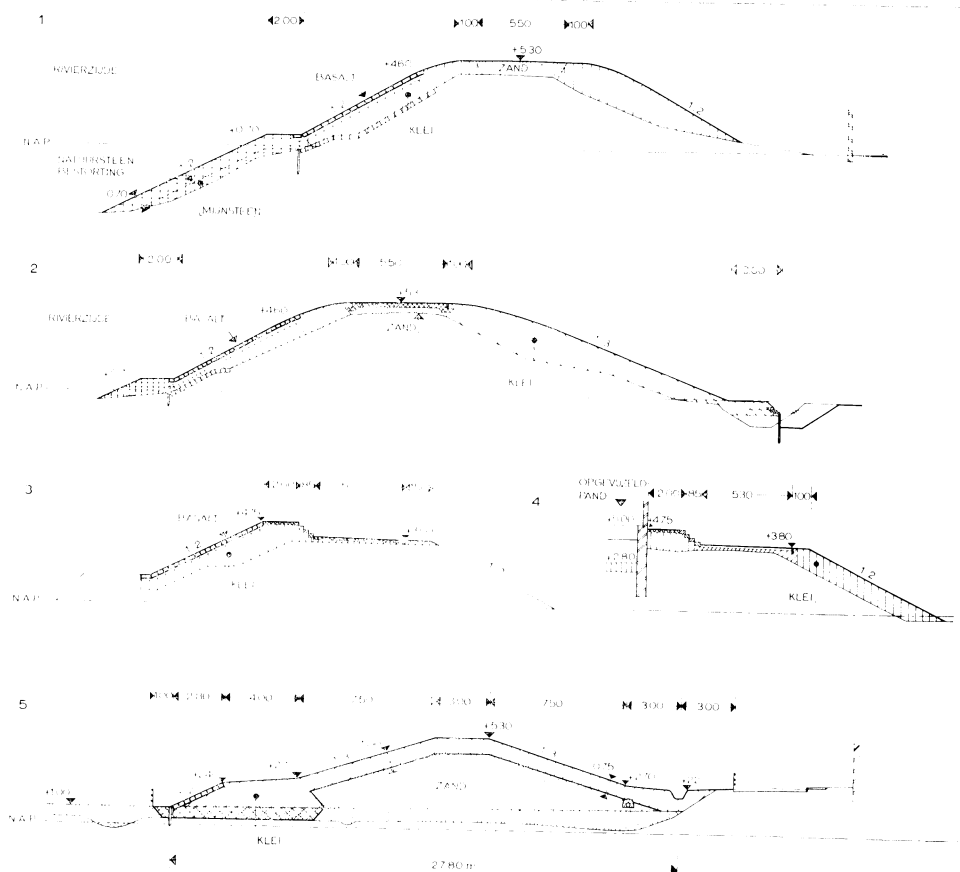
Dwarsprofielen van de dijkverhoging
