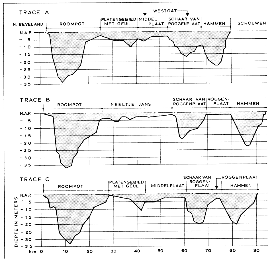
DWARSPROFIELEN WESTELUKE TRACEZONE
