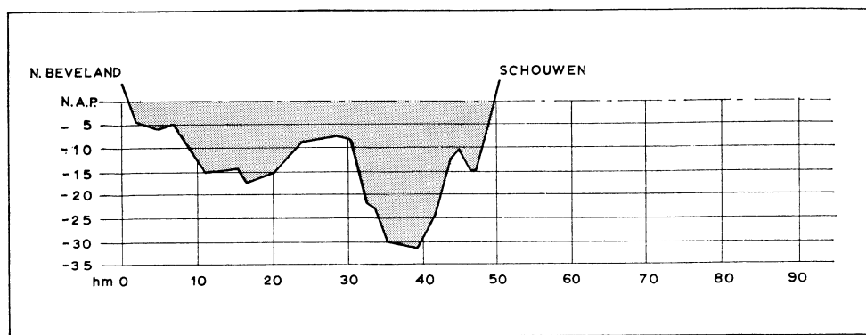
VOORBEELD VAN EEN DWARSPROFIEL OOSTELUKE TRACEZONE
