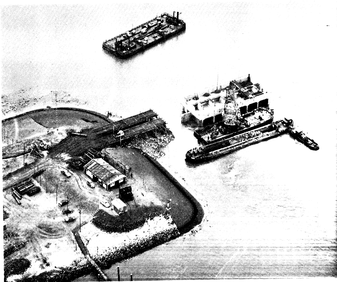
Aansluiting van de eerste caisson op het landhoofd
