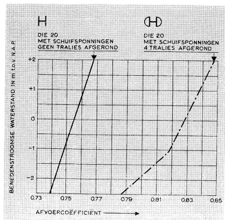
Afvoercoëfficiënt van de caissons
