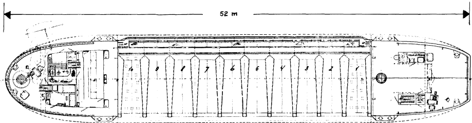
Lengtedoorsnede en bovenaanzicht van de 'Lauwerszee'
