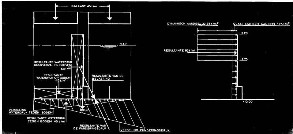
Geschematiseerde verdeling van de statische, de quasi-statische en de dynamische belastingen op de caissons
