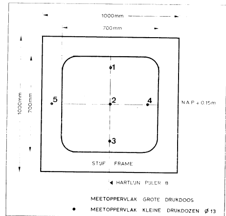
Overzicht van een gedeelte van de apparatuur die gebruikt wordt bij de pulsatie- en excitatiemetingen
