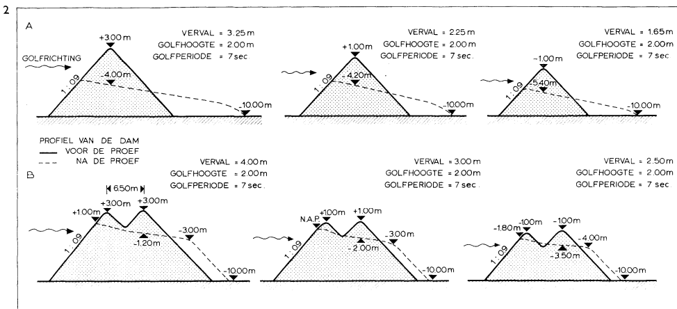
Fig. 2. Vervorming van een uit betonblokken opgebouwde dam met enkele en dubbele kruin onder invloed van stroom en golven uit dezelfde richting
