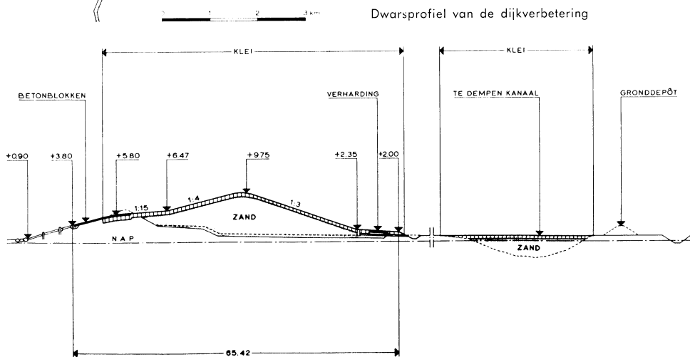
Dwarsprofiel van de dijkverbetering
