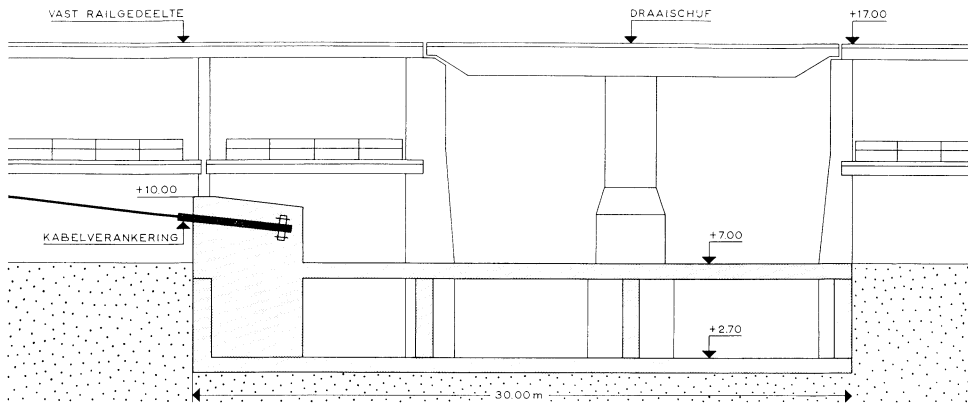
De vaste verankering op de Middelpilaar
