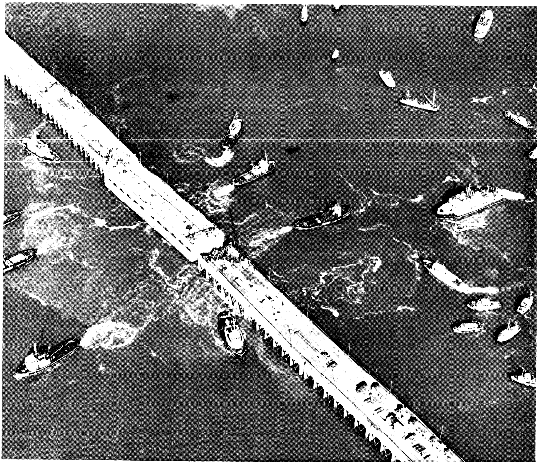
Het indraaien van de laatste twee, aan elkaar gekoppelde, caissons
