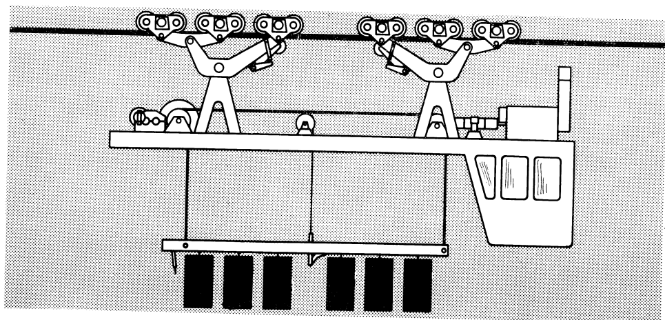
Schets van het nieuwe type motorgondel
