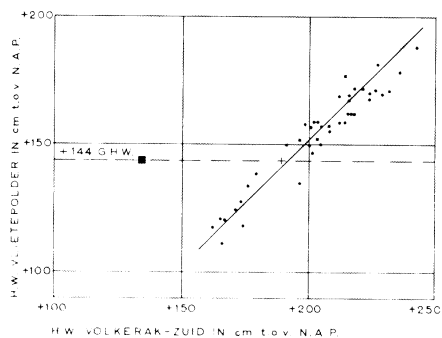
3-6. Correlatie tussen de registraties van de H.W.- en L.W.-standen in de stations Volkerak-zuid, Steenbergse Sas, Bruinisse en Stavenisse enerzijds en het station Vlietepolder in de Oosterschelde anderzijds
