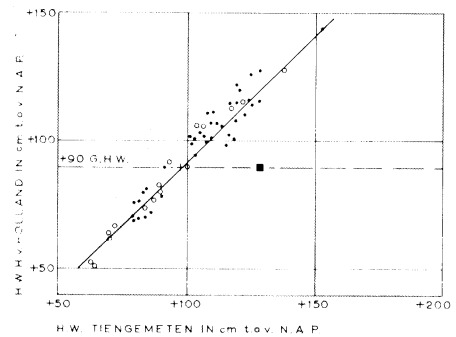
7-8. Correlatie tussen de registraties van de H.W.- en L.W.-standen in de stations Tiengemeten en Moerdijk enerzijds en het station Hoek van Holland anderzijds
