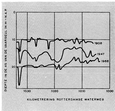
Fig. 24. Het diepteverloop van de Rotterdamse Waterweg in verschillende perioden
