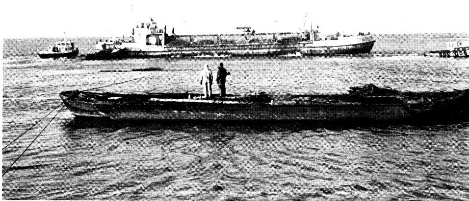
Het stuk wordt bestort. Op de voorgrond de bak die dient voor het in de goede richting houden van het stuk
