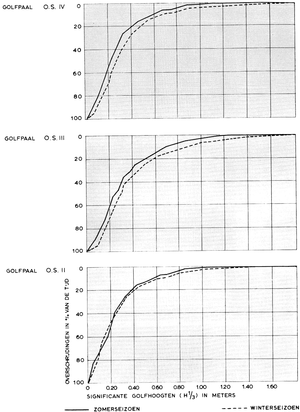
Fig. 4. Overschrijdingsfrequenties van significante golfhoogten
